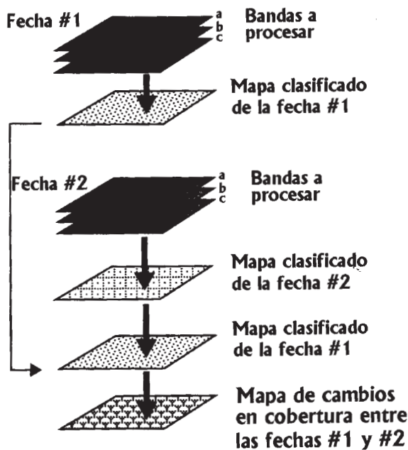
FIGURA 24.9 Esquema generalizado para detectar un cambio en la cobertura (p.ej., etapas sucesionales del bosque) a partir de una secuencia temporal de imágenes espectrales. Es importante aclarar que la resolución temporal puede aumentarse añadiendo fechas y/o reduciendo el intervalo de tiempo entre fechas. Este mismo esquema aplica a imágenes pancromáticas (fotos aéreas en blanco y negro), pero habría que reducir el número de bandas utilizadas a una sola.
