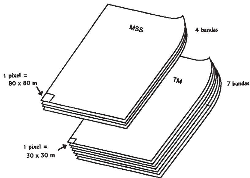
FIGURA 24.4 Diagrama que compara algunas características de los datos obtenidos por instrumentos Landsat MSS y Landsat TM. El tamaño de los cuadrados que ilustran un píxel de cada escena se ha exagerado. Como se ve, los datos Landsat varían en resolución espacial y resolución espectral, pero poseen el mismo ancho y largo de escena (ver Tabla 24.1; modificado de ERDAS 1991)
