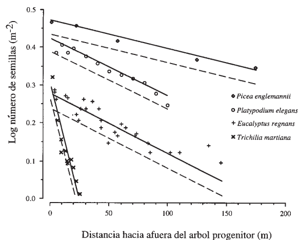
FIGURA 15.2 Curvas de dispersión de semillas, ajustadas estadísticamente, para cuatro especies de árboles: Trichilia , Eucalyptus , Platypodium y Picea (según Dirzo & Domínguez 1986). La línea punteada representa la curva de dispersión esperada en condiciones de depredación previa a la dispersión (se espera una reducción de un 50 % en la producción de semillas) y suponiendo que no hay cambios en el índice de visitación de los dispersores. Si la producción de semillas se reduce en un 50%, las especies estudiadas presentarían la siguiente reducción en sus patrones de dispersión espacial: Trichilia , hasta 3 m, Eucalyptus , hasta 19 m, Platypodium , hasta 19 m, y Picea , hasta 48 m.
