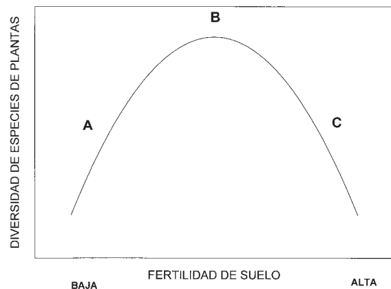
FIGURA 9.1 Modelo que muestra una posible relación entre la diversidad de plantas de una comunidad “madura” y la fertilidad del suelo (basado en Huston 1997). Pocas especies pueden adaptarse a un ambiente poco fértil; en un ambiente muy fértil los mejores competidores desplazan a sus rivales. Nótese que para apreciar la relación es importante evaluar todo el gradiente de condiciones. Los datos de la región A indican una correlación positiva entre la diversidad de plantas y la fertilidad del suelo, en la región B tal relación no existe, y en la región C se trata de una correlación negativa. Estas relaciones podrían verse alteradas por la presencia de una perturbación, lo cual detendría el proceso de exclusión competitiva en la región C y abriría nuevos nichos en la comunidad. Para evaluar este modelo hipotético se necesitarían datos representativos sobre la diversidad de plantas, los nutrientes del suelo, y el efecto de las perturbaciones a lo largo de un amplio gradiente de condiciones ecológicas.
