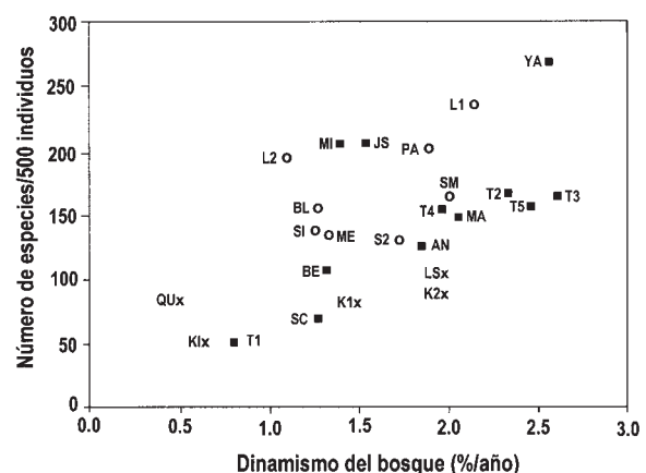
FIGURA 16.1 Riqueza de especies de árboles en función del dinamismo del bosque (media de mortalidad y reclutamiento anual). Cada punto representa un bosque húmedo, o un bosque lluvioso en una determinada localidad tropical. Modificado de Phillips et al. (1994).
