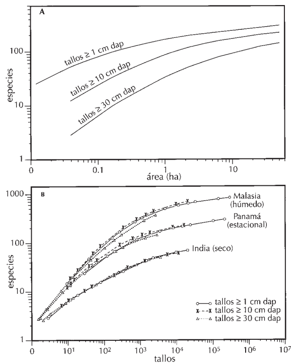
FIGURA 4.2 A. Curvas de número de especies por área para tres clases de diámetro a la altura del pecho (d.a.p.) en una parcela de 50 hectáreas en la Isla de Barro Colorado, en Panamá. B. Curvas de número de especies por individuo para tres parcelas de 50 hectáreas en distintas localidades. Nótese que las curvas de diferentes clases de diámetro de árboles en cada parcela son esencialmente las mismas, pero la diversidad global aumenta considerablemente desde la parcela más seca hasta la más húmeda. Es por esto que una manera de comparar la diversidad de especies entre sitios o muestras es basándose en el número de individuos, independientemente del área. Adaptado de Condit et al. (1998).
