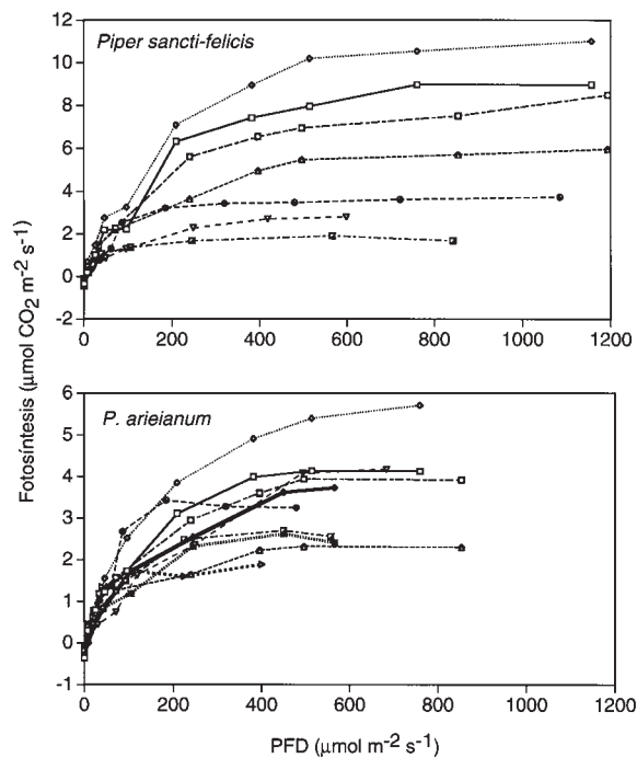
FIGURA 10.1 Curvas de respuesta fotosintética a la luz. Para el estudio se utilizaron estacas de Piper sancti-felicitis y de P. arieianum plantadas en macetas y colocadas a lo largo de diversos transectos en los claros de un bosque lluvioso en Costa Rica. Ambas especies fueron expuestas al mismo ámbito de condiciones de luz, y aunque ambas dieron muestras de plasticidad en su respuesta fotosintética, P. sancti-felicitis mostró una mayor capacidad fotosintética. PFD= densidad de flujo de fotones.
