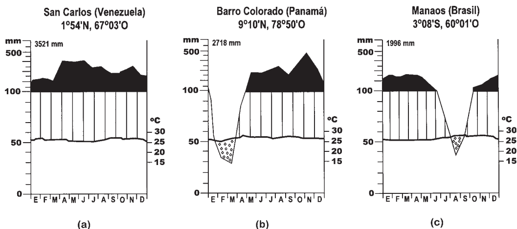
FIGURA 7.1 Climadiagramas de estaciones en bosques húmedos y lluviosos neotropicales. El climadiagrama de San Carlos de Río Negro (Venezuela), representa el patrón uniforme de lluvias, y el de la Isla de Barro Colorado (Panamá) y Manaus (Brasil) el unimodal, al norte y sur del ecuador climático, respectivamente. Adaptado de Walsh (1996). La parte negra en los climadiagramas representa la precipitación media mensual por encima de los 100 mm y se interpreta como un “exceso” de agua. La parte punteada representa meses “secos” en los que la evapotranspiración supera las entradas por precipitación.
