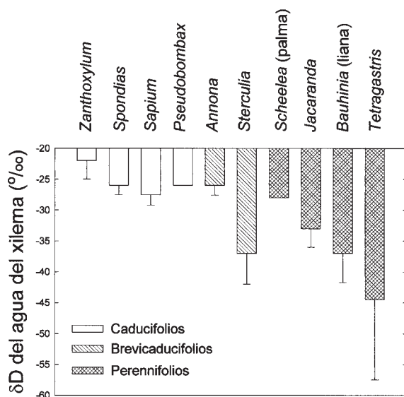
FIGURA 11.3 Contenido relativo de isótopos estables de hidrógeno ( \delta D ) en el agua del xilema de un grupo de especies caducifolias, breviducifolias y perennifolias. Los datos provienen de un bosque húmedo localizado en la península de Gigante, en las cercanías de la Isla de Barro Colorado, Panamá. Las muestras de agua se obtuvieron al finalizar la estación seca de 1992. Las líneas verticales debajo de las barras indican el error estándar (adaptado de Jackson et al. 1995).
