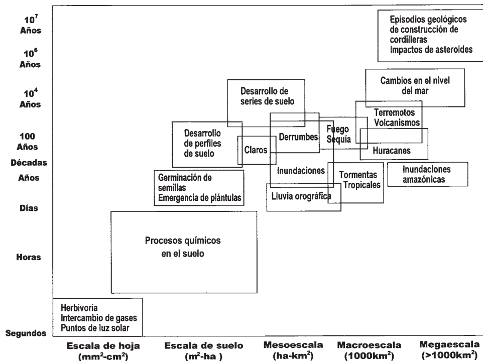
FIGURA 1.3 Perturbaciones naturales en función de su escala de acción y de su intervalo temporal de retorno (frecuencia) en los ecosistemas terrestres, particularmente en los bosques húmedos y lluviosos neotropicales. (El término “puntos de luz solar” que aparece en el primer rectángulo equivale al término “destellos de luz”, descrito en los capítulos 6 y 10.)
