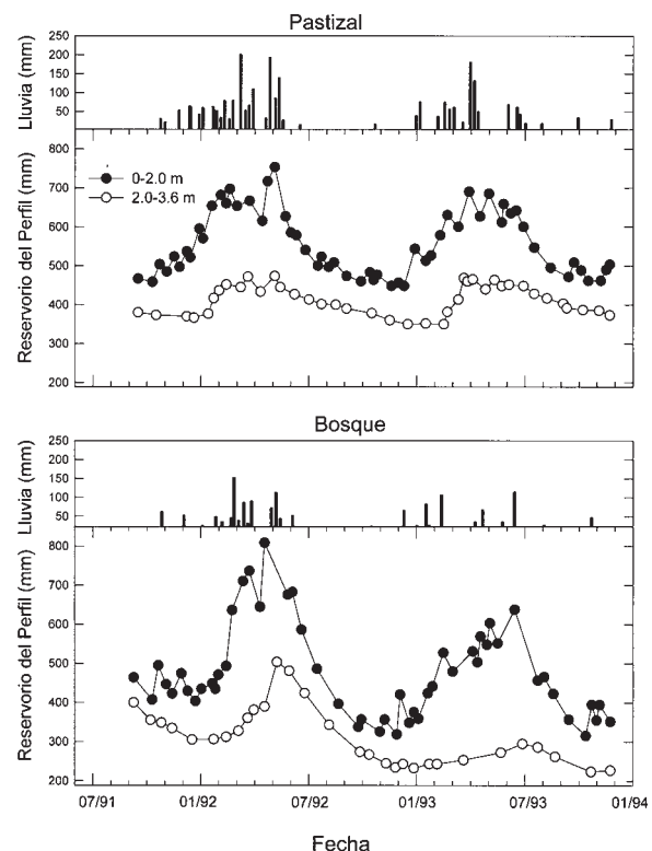
FIGURA 7.4 Lluvias y reservorios de agua en el perfil del suelo en dos horizontes (0-2.0 m y 2.0-3.6 m) bajo pastizales (Fazenda Boa Sorte; 5° 10' S; 48° 45' W) y bosques (Reserva Vale do Rio Doce; 5° 45' S; 49° 10' W) en Marabá, Pará, Brasil. Modificado a partir de Hodnett et al. (1996).
