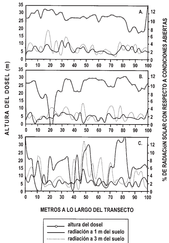
FIGURA 6.5 Relación entre estructura del bosque (altura del dosel) y ambiente lumínico medido a 1 y 3 m sobre el piso y a lo largo de tres transectos de 100 m en el bosque primario de la Estación Biológica La Selva, en Costa Rica. Transectos con un coeficiente de variación de la altura bajo (A: 14%), intermedio (B: 27%) y alto (C: 60%). Modificado de Clark et al. (1996).
