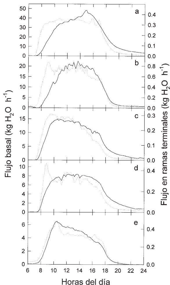
FIGURA 11.4 Flujo diario de agua observado en las ramas terminales (líneas punteadas) y en la base del tronco (líneas sólidas) de los siguientes árboles: (a) Anacardium excelsum , (b) Ficus insipida , (c) Luehea seemannii , (d) Spondias mombin , y (e) Cecropia longipes , durante algunos días que se consideraron representativos de la estación seca de 1996. Bosque del Parque Metropolitano de Panamá (adaptado de Goldstein et al. 1998).
