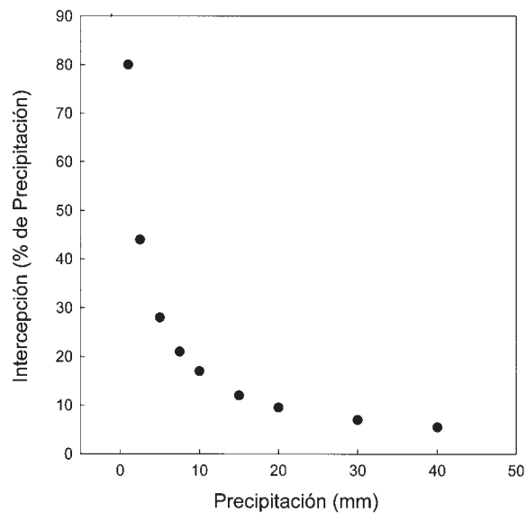
FIGURA 7.3 Relación entre la pérdida de agua por intercepción y el volumen de lluvia de aguaceros individuales en un bosque montano en Tanzania. Datos tomados de Jackson (1971).
