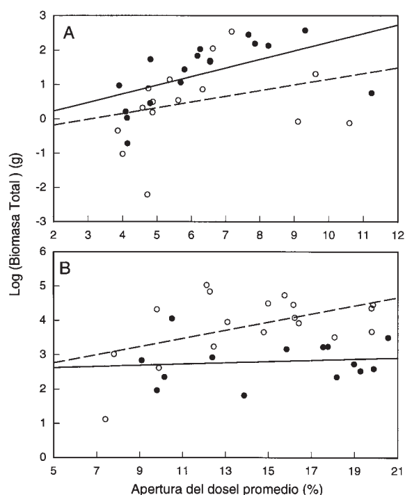
FIGURA 10.4 Crecimiento de la biomasa de las estacas de Piper sancti-felices (o) y P. arieianum (•), 13 meses después de haber sido colocadas en (A) un claro pequeño (52 m 2 ), y (B) en un claro grande (300 m 2 ). Con base en el análisis de tres grupos de fotografías hemisféricas tomadas durante el experimento, se observó que en el claro pequeño sólo la biomasa de P. arieianum mostró una dependencia significativa en función de la apertura promedio del dosel. En el claro grande, sólo P. sancti-felices mostró una respuesta de crecimiento significativa a la apertura promedio del dosel.
