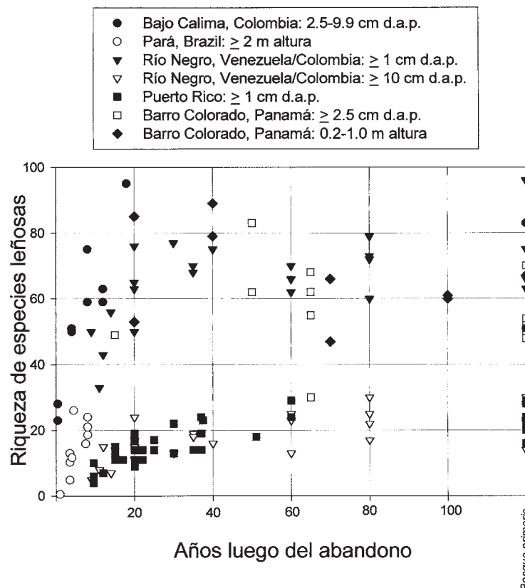
FIGURA 23.5 Acumulación de riqueza de especies leñosas durante la sucesión secundaria (en contraste con lo encontrado en un bosque primario). Los datos contemplan diferentes localidades neotropicales de baja, húmedas y lluviosas, en las que el uso de la tierra previo al abandono del sitio había sido de leve a moderado. Las fuentes citadas son: Bajo Calima: Faber-Langendoen (1992); Pará: Uhl et al. (1988); Río Negro: Saldarriaga et al. (1988); Puerto Rico: Aide et al. (1996), Rivera y Aide (1998); Barro Colorado: Knight (1975), para troncos ≥ 2.5 cm d.a.p.; Denslow y Guzmán (2000). Debido a diferencias, tanto en el área de muestreo como en las clases de tamaño estudiadas, las tendencias en el tiempo deben analizarse para un mismo estudio y no entre estudios diferentes.
