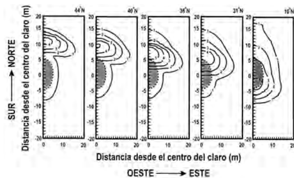
FIGURA 6.3 Efecto de la latitud sobre la distribución espacial de la luz dentro y fuera de los claros producidos por la caída de árboles. El área del claro es definida por la línea discontinua (---) y aparece sombreado de color gris. Las líneas continuas indican la cantidad de luz incidente (en una escala ascendente de 1 a 5). Los gráficos corresponden a diferentes bosques en la zona templada (44°N, 40°N, 36°N y 31°N) y a un bosque tropical de bajura (10°N). Nótese que en las latitudes altas, la mayor cantidad de radiación incidente no cae en el centro del claro sino hacia el norte del mismo, mientras que en el trópico, la mayor cantidad de radiación incidente cae en el centro del claro y es espacialmente más uniforme. Modificado de Canham et al. (1990).
