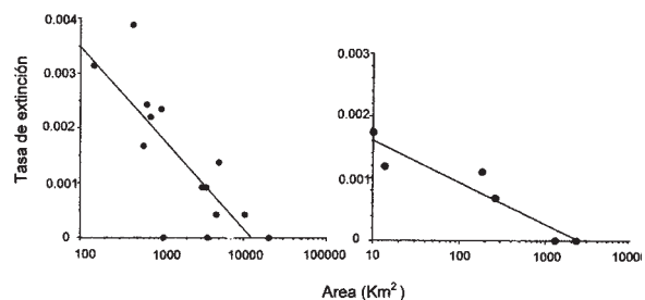
FIGURA 22.2 Extinción de mamíferos en parques nacionales de Norte América y Tanzania, documentada desde la creación y aislamiento del parque. La tasa de extinción fue medida por un parámetro definido como dS/dt = -kS , donde S = número de especies y dS/dt es el cambio de S por unidad de tiempo. Nótese que incluso los parques más grandes (10 000 km 2 ) pueden perder especies después de ser aislados (modificado de Newmark 1995, 1996).
