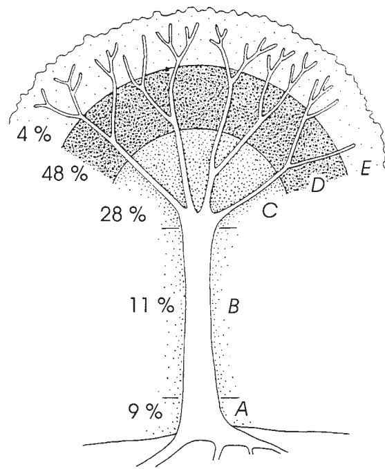
FIGURA 12.2 Distribución idealizada de las especies de orquídeas epífitas presentes en los árboles de un bosque lluvioso en África. Los números a la izquierda indican el porcentaje de especies que se encuentra en una zona particular del árbol. (A) es la parte basal del tronco hasta 3 m por encima del suelo, (B) es el tronco hasta la primera ramificación, y (C), (D) y (E) son secciones de la copa, la cual fue dividida en tres partes iguales (modificado de Johansson 1974).
