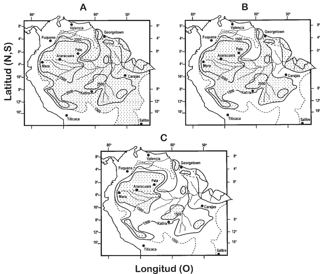
FIGURA 2.4 Distribución (simplificada) del bosque húmedo y lluvioso neotropical de bajura en Suramérica, en función de las isoyetas correspondientes a 2 500 mm, 2 000 mm y 1 500 mm de precipitación (precipitación actual) (A), luego de una reducción de 25% en la precipitación actual (B), y luego de una reducción de 40% en la precipitación actual (C). El escenario C concuerda con los datos palinológicos de la región durante el Pleistoceno: presencia de bosques en Mera, Araracuara y Pata, y presencia de vegetación de sabana en Katira, Carajas y Georgetown. Modificado de Van der Hammen y Absy (1994) y Hooghiemstra y Van der Hammen (1998).
