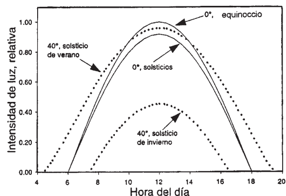
FIGURA 6.2 Intensidad relativa de la luz solar, según la hora del día, en diferentes latitudes.
