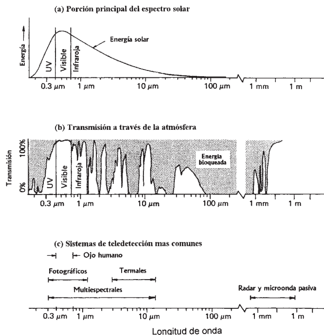
FIGURA 24.1 Características espectrales de: (a) la porción principal del espectro solar, (b) los efectos atmosféricos, y (c) los sistemas más comunes de teledetección. (Modificado de Lillesand & Kiefer 1994.)
