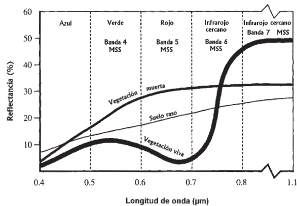
FIGURA 24.6 Respuesta espectral de la vegetación verde, de la vegetación muerta y del suelo desnudo, según las bandas del espectro electromagnético detectadas por los sensores del satélite Landsat MSS. Nótese que las principales diferencias en respuesta espectral entre los objetos ilustrados se dan en las porciones roja e infrarroja cercana. (Modificado de Jensen 1996.)
