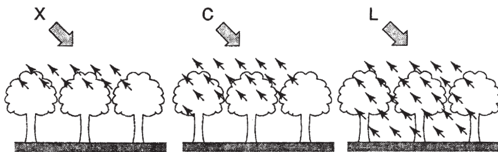
FIGURA 24.8 Interacción de las radiaciones emitidas por los sistemas de radar en las bandas X, C, y L. Las longitudes de onda aumentan desde la banda X a la banda L; por lo tanto, los factores que controlan la retrodispersión cambian desde los componentes del dosel –en la banda X– hasta los troncos y el suelo –en la banda L–. Las flechas anchas indican la dirección de la señal emitida desde el instrumento de radar, mientras que las flechas estrechas indican la dirección de retrodispersión. (Modificado de Foody & Curran 1994.)
