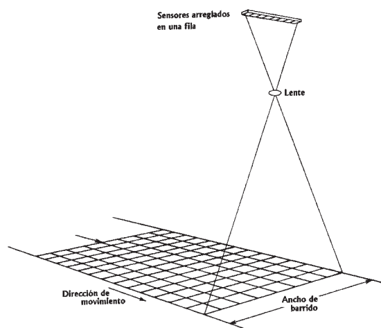
FIGURA 24.3 Diagrama simplificado de la adquisición de datos teledetectados mediante barrido. El lente y la fila de sensores ilustrados estarían dentro del instrumento sensor, y éste, a su vez, estaría colocado en un avión o un satélite. El diagrama muestra una fila de sensores con ocho elementos. (Modificado de Lillesand & Kiefer 1994.)
