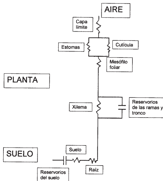
FIGURA 11.1 Vías de circulación del agua. Se incluyen los puntos que presentan mayor resistencia hidráulica (representados como resistencias eléctricas en serie) y los reservorios de agua en el suelo y en los tallos (representados como capacitores). En la hoja, las resistencias cuticulares y estomáticas se representan como resistencias paralelas.
