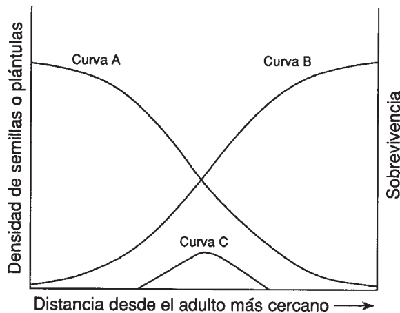
FIGURA 19.3 El modelo de Janzen y Connell como una posible explicación del mantenimiento de la diversidad de árboles en los bosques tropicales. La Curva A representa la cohorte de semillas o de plántulas producida por un árbol adulto. La Curva B es la curva de sobrevivencia y muestra cómo la sobrevivencia de las semillas y de las plántulas aumenta conforme aumenta la distancia del adulto coespecífico más cercano. La Curva C es la curva de reclutamiento y señala que la probabilidad de reclutamiento debería alcanzar su máximo a distancias intermedias, o sea, en aquellos sitios en donde todavía hay bastantes semillas o plántulas pero donde también existe cierta probabilidad de sobrevivencia. Este patrón de reclutamiento se reflejaría en un “espaciamiento” de los árboles adultos de cualquier especie del bosque. De acuerdo con Janzen y Connell, es posible que los árboles adultos actúen como un “reservorio” de enemigos naturales (patógenos, herbívoros), los cuales podrían atacar a las semillas y plántulas que se encuentran más cercanas al árbol progenitor. En otros capítulos se hace referencia al patrón espacial sugerido por Janzen y Connell, no desde el punto de vista del herbivorismo per se , sino desde la perspectiva de los patógenos (capítulo 18) y los depredadores de semillas (capítulos 15 y 16). Adaptado de Janzen (1970).
