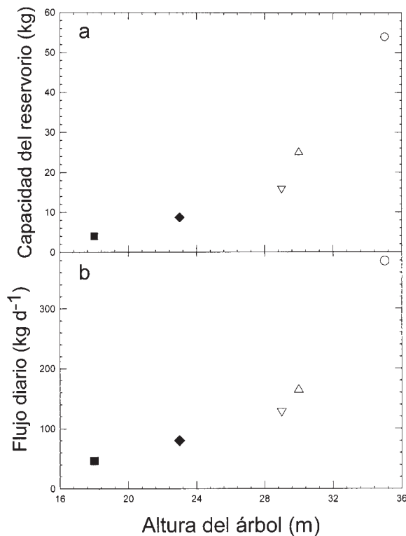
FIGURA 11.5 Relación entre (a) la capacidad diaria de los reservorios internos (en kg de agua) y la altura de los árboles, y (b) el flujo diario de savia y la altura de los árboles. Los puntos representan las mismas especies que aparecen la Figura 11.4 (adaptado de Goldstein et al. 1998).
