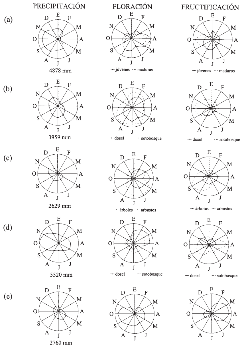
FIGURA 17.1. Patrones anuales de precipitación, floración y fructificación en cinco sitios de bosque lluvioso de baja en el neotrópico. (a) Los Tuxtlas, México, 22 especies de árboles, se registraron flores y frutos en estado joven y maduro (Carabias-Lillo & Guevara 1985). (b) Estación Biológica La Selva, Costa Rica, 93 especies de árboles del dosel y 92 especies de árboles del sotobosque (Frankie et al. 1974). (c) Isla de Barro Colorado, Panamá, 365 especies de árboles y 93 especies de arbustos (Croat 1969, 1975). (d) Alto Yunda, Colombia, 164 especies de árboles (Hilty 1980). (e) Reserva Forestal 'His/Her Majesty Penal Settlement', Guyana, 190 especies de árboles (ter Steege & Persaud 1991). En las gráficas de precipitación, los ejes radiales representan un intervalo de 800 mm.
