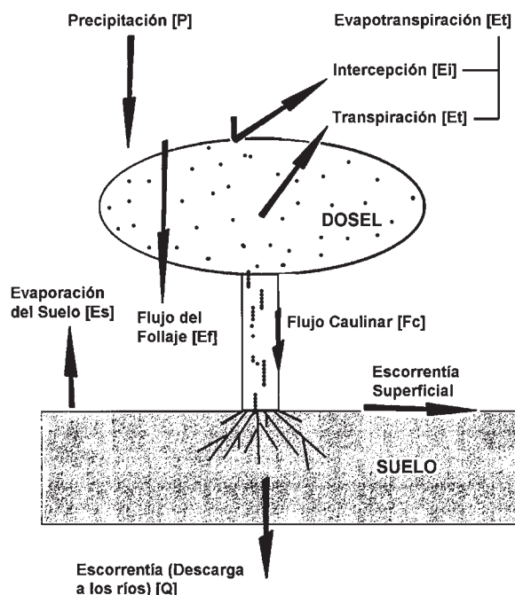
FIGURA 7.2 Representación de los flujos más importantes del balance hídrico en un bosque.
