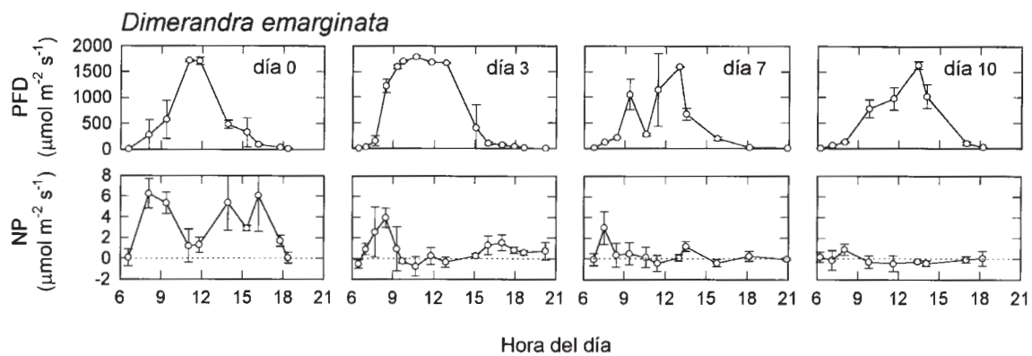
FIGURA 12.3 Cambios observado in situ en el intercambio neto de CO 2 (NP) entre la orquídea epífita Dimerandra emarginata y la atmósfera durante un período de sequía en Panamá. En el gráfico aparecen la densidad de flujo de fotones (PFD) y el NP antes de comenzar la sequía (día 0) y luego de haber comenzado ésta (días 3, 7 y 10). Los valores representan promedios \pm 1 desviación estándar (modificado de Zotz y Tyree 1996).
