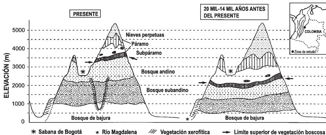
FIGURA 2.1 Distribución altitudinal de la vegetación de los Andes orientales de Colombia, en la actualidad y durante la última glaciación (unos 18 mil años antes del presente). Los cambios altitudinales responden, principalmente, a variaciones en la temperatura ambiental. Durante la última glaciación, la Sabana de Bogotá (2 500 m.s.n.m.) estaba rodeada de vegetación de páramo; actualmente, se encuentra rodeada de bosque montano alto. Modificado de Van der Hammen (1974) y Hooghiemstra y Cleef (1995).
