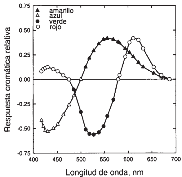
FIGURA 6.7 Modelo de la percepción de colores por los seres humanos, basado en el concepto de dos sistemas diferentes que contrastan el amarillo con el azul, y el verde con el rojo. Cada línea en la gráfica representa uno de los contrastes. La respuesta cromática relativa indica la intensidad con la cual se estimula el contraste. Por ejemplo, una longitud de onda de 550 nm estimula el amarillo del contraste amarillo-azul, y el verde del contraste verde-rojo. Como resultado, esta longitud de onda es percibida por los humanos como un verde brillante. En cambio, una longitud de onda de 625 nm estimula las respuestas amarillo y rojo y es percibido como un anaranjado. Modificado de Hurvich (1981).
