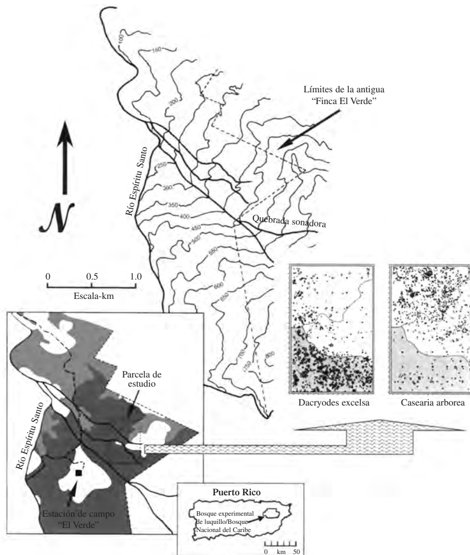
FIGURA 5.3 Uso de la tierra en la antigua “Finca El Verde”, Puerto Rico, en 1934, momento en que la parcela fue adquirida por el Servicio Forestal de los Estados Unidos. El color gris claro del mapa indican áreas que fueron totalmente deforestadas. El color blanco indica áreas medianamente taladas y el color gris oscuro indica áreas que no fueron taladas, pero que fueron afectadas por el cultivo del café y otros usos de la tierra. También se incluye la distribución de las especies de árboles Dacryodes excelsa y Casearia arborea en una parcela de estudio de 16 hectáreas (modificado de Willig et al. 1996).
