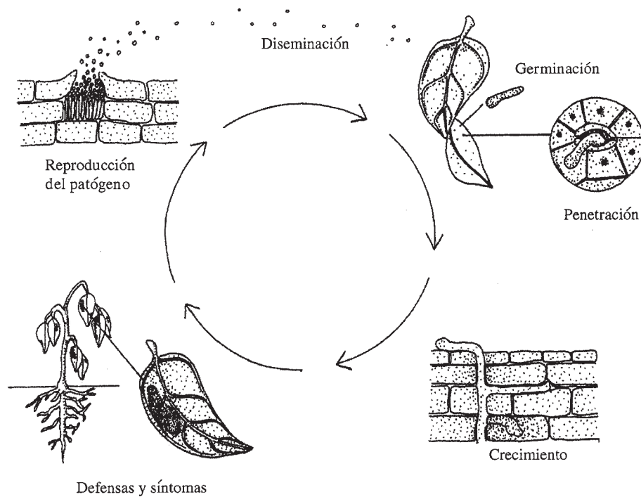
FIGURA 18.4 Ciclo de vida de una enfermedad vegetal típica. Dicho ciclo supone: diseminación, germinación de esporas, penetración y crecimiento a través del hospedero, respuesta del hospedero y reproducción del patógeno.
