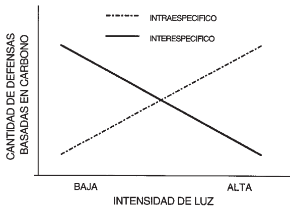
FIGURA 19.4 Variaciones intra-específicas e inter-específicas de las defensas basadas en carbono. Dada una especie, y en virtud de una mayor luminosidad, se observa que las plantas invierten el exceso de carbono fijado durante la fotosíntesis en la producción de defensas. Dada una serie de especies diferentes, se verá que las plantas que se encuentran en los hábitats más iluminados crecerán más rápidamente e invertirán menos en defensas, incluso en defensas basadas en carbono. Para más detalles ver Recuadro 19.2.
