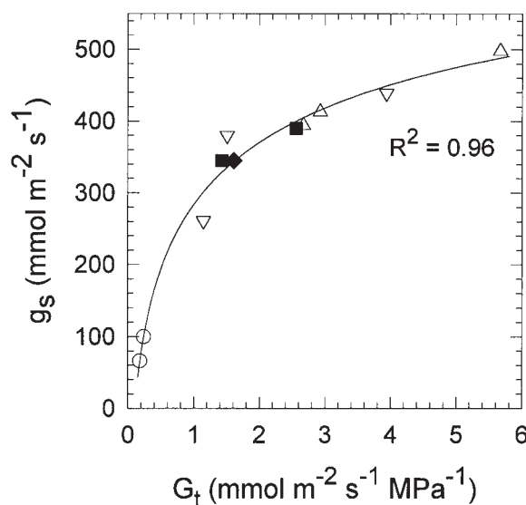
FIGURA 11.7 Relación entre conductancia estomática g_s y conductancia hidráulica total G_t observada en cuatro especies de un bosque húmedo de Panamá. Los símbolos corresponden a los de la Fig. 11.5 (adaptado de Andrade et al. 1998).
