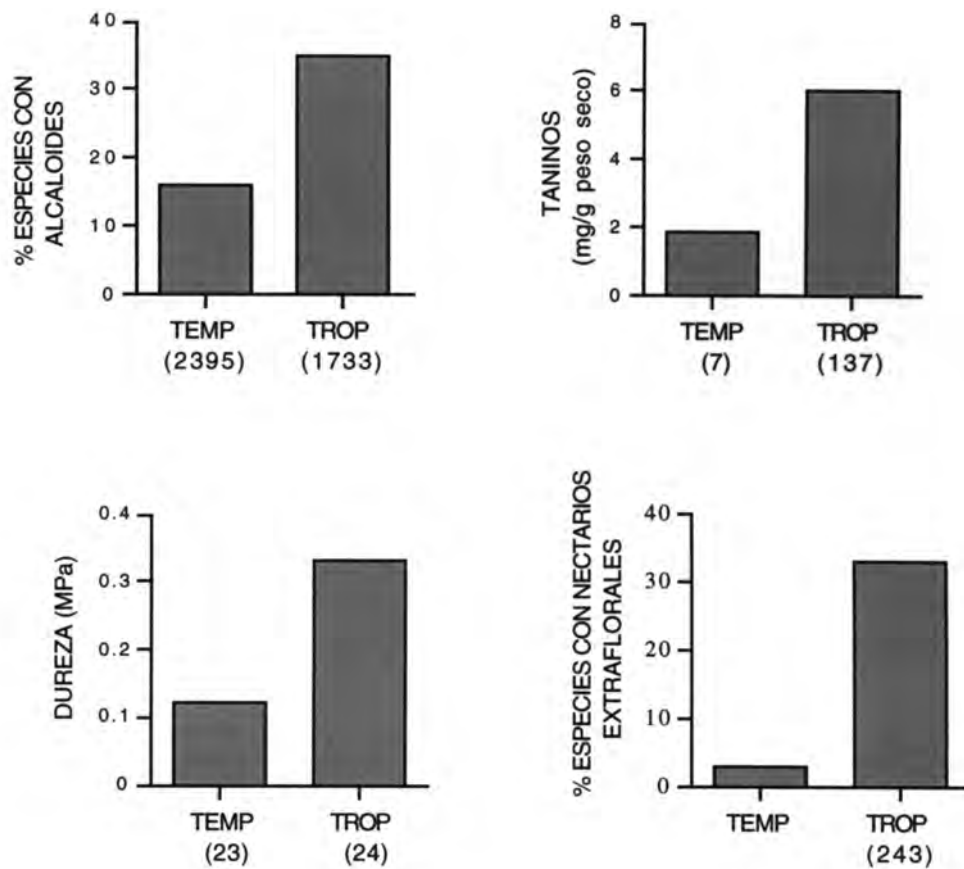
FIGURA 19.1 Nivel de defensas vegetales. Comparación latitudinal: a) porcentaje de especies con alcaloides; b) concentración de taninos condensados en hojas maduras extraídos con BuOH/HCl; c) dureza de las hojas maduras medida como la fuerza necesaria para perforar una hoja (en MegaPascuales); d) porcentaje de especies con nectarios extraflorales en las hojas jóvenes. Entre paréntesis aparece el número de especies de las que se tenía información. Los datos son de Coley y Aide (1991).
