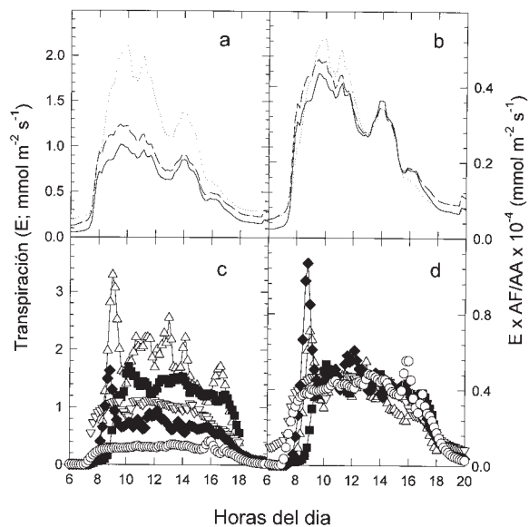
FIGURA 11.6 A y B: Variación en la tasa de transpiración diurna de tres ramas terminales de Luehea seemannii (sin normalizar) y variación normalizada por la razón área foliar (AF): área de la albura (AA) de las ramas. C y D: Variación en la tasa diurna de transpiración de 4 especies de un bosque húmedo panameño (sin normalizar) y variación normalizada por la razón AF: AA (ver texto). Los símbolos corresponden a los de la Fig. 11.5 (adaptado de Andrade et al. 1998).
