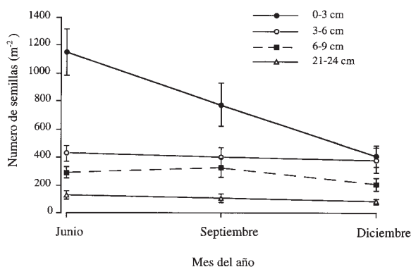
FIGURA 15.4 Densidad media del banco de semillas ( \pm 1 error estándar) en el bosque de la Isla de Barro Colorado, Panamá. Las mediciones se efectuaron en 1993 a cuatro profundidades distintas y en tres períodos diferentes (según Dalling et al. 1997b).
