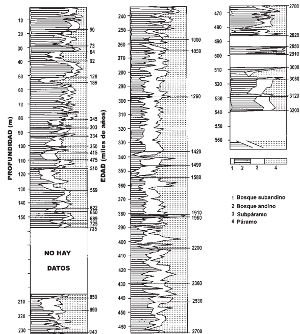
FIGURA 2.2 Diagrama de deposición de polen en una muestra de 586 m de profundidad (representando entre 3.2 millones de años y 27 mil años antes del presente), proveniente de la Sabana de Bogotá, Colombia. La estimación de la edad de cada estrato se fundamentó en el análisis de las cenizas volcánicas y en calibraciones basadas en la proporción de oxígeno isotópico presente en la atmósfera en un período determinado. Se observa la variación en la contribución relativa (eje horizontal), dada una misma elevación, del polen de cuatro comunidades vegetales: bosque subandino (montano bajo), bosque andino (montano alto), subpáramo y páramo. Modificado de Hooghiemstra y Ran (1994).
