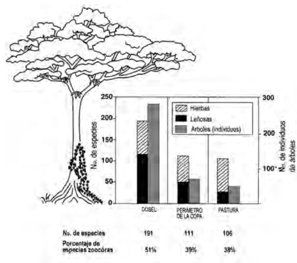
FIGURA 23.2 Formas de crecimiento identificadas en una muestra de 256 árboles remanentes en pasturas, en tres microhábitats, en la región de Veracruz, México. La escala de la derecha cuantifica el número de individuos de especies arbóreas encontradas en la muestra. La escala de la izquierda cuantifica el número de especies herbáceas y leñosas (incluye árboles). Para cada microhábitat se presenta el porcentaje de especies cuyas semillas son dispersadas por animales. Modificado de Guevara et al. (1992).
