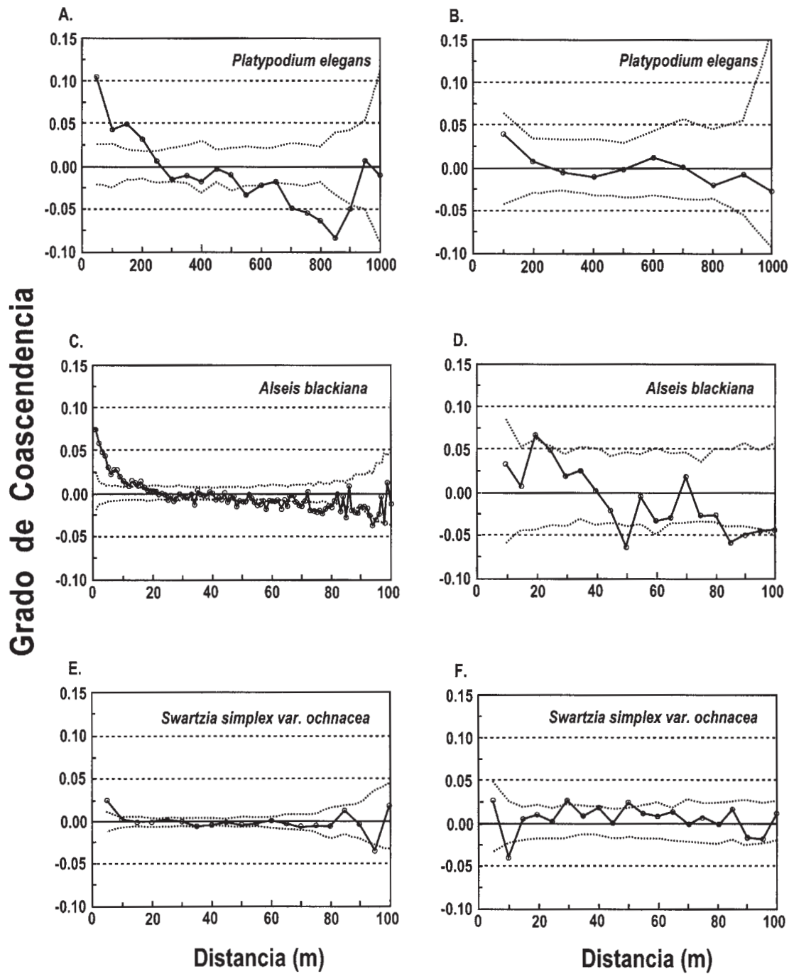
FIGURA 13.2 Grado de ascendencia común o grado de autocorrelación genética (valores del eje y) en tres especies de árboles en el bosque de la Isla de Barro Colorado en Panamá. Los estimados se obtuvieron a partir de varios loci y se representan gráficamente en función de la distancia entre parejas de individuos. Los círculos abiertos representan la ascendencia común media estimada en intervalos de distancia sucesivos y la línea punteada indica un intervalo de confianza del 96%, generado por métodos de remuestreo o “bootstrap” a partir de la hipótesis nula de que no existe ninguna similitud en la información genética entre pares de individuos (valor de ascendencia común = 0). (A) y (B): Platypodium elegans , individuos de 1-2 cm y > 15 cm de diámetro a la altura del pecho (d.a.p.), respectivamente. (C) y (D): Alseis blackiana , individuos de 1-2 cm y > 15 cm d.a.p., respectivamente. (E) y (F): Swartzia simplex var. ochracea , individuos menores a 1 cm y mayores a 5 cm de d.a.p., respectivamente. La historia natural de estas especies se describe en el texto y en el Recuadro 13.5.
