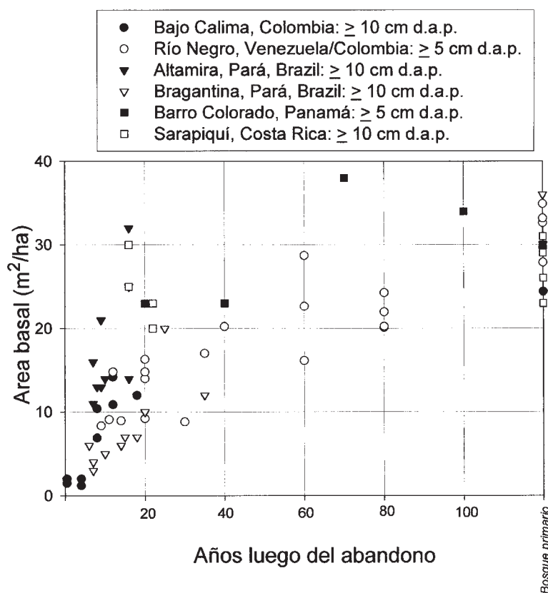
FIGURA 23.4 Acumulación de área basal durante el proceso de sucesión secundaria. Los datos contemplan diferentes localidades neotropicales de bajura, húmedas y lluviosas, en las que el uso de la tierra previo al abandono del sitio había sido de leve a moderado. Las fuentes citadas son: Bajo Calima (Entisoles): Faber-Langendoen (1992); Río Negro (Oxisoles antiguos): Saldarriaga et al. (1988); Altamira (Alfisoles): Tucker et al. (1998); Bragantina (Oxisoles antiguos): Tucker et al. (1998); Barro Colorado (Oxisoles y Alfisoles recientes): Denslow y Guzmán (2000); Sarapiquí (Ultisoles e Inceptisoles): Guariguata et al. (1997), Guillén (1993), Lieberman y Lieberman (1994).
