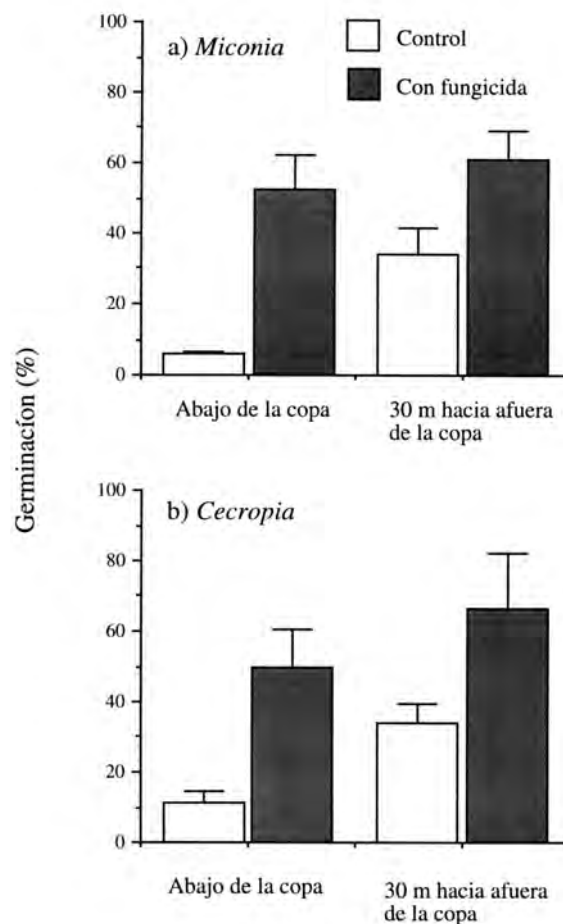
FIGURA 15.5 Germinación promedio (indicativa de la viabilidad de las semillas) luego de seis meses de enterramiento (+ 1 error estándar). Isla de Barro Colorado, Panamá. Se trabajó con dos grupos de semillas de árboles pioneros, a uno se le aplicó fungicida y el otro se dejó tal cual. Las semillas se introdujeron en bolsas de nylon semipermeables y se enterraron, unas bajo la copa del árbol y otras a 30 m del individuo adulto coespecífico más cercano (según Dalling et al. 1998).
