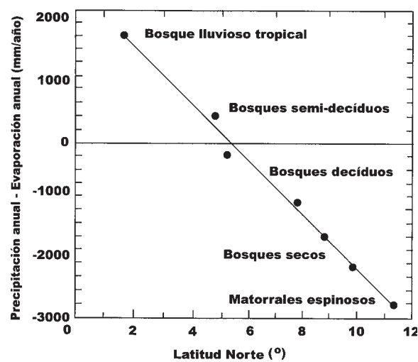
FIGURA 1.2 Principales tipos de bosque de Venezuela a lo largo de un gradiente latitudinal y en función de la diferencia entre precipitación y evaporación. Modificado de Medina (1983).
