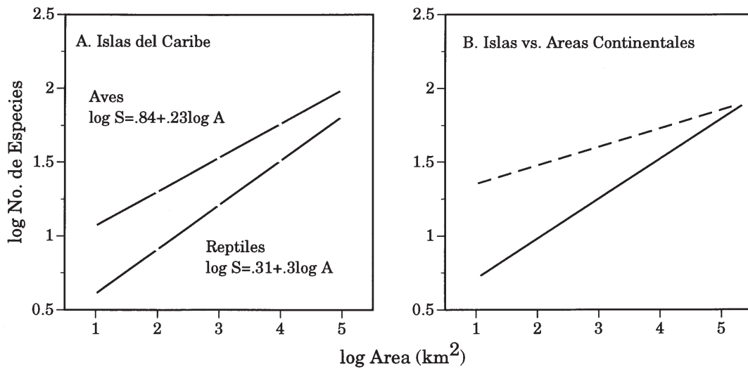
FIGURA 22.1 A. Relación entre el área y el número de especies de aves y reptiles (S) en las islas del mar Caribe (modificado de Wright 1981). B. Relación entre el área y el número de especies en un archipiélago (línea continua) y en áreas similares en el continente (línea punteada). Posiblemente debido a la naturaleza de la matriz, para una misma área el continente tiene más especies que la isla (modificado de Holt 1993).
