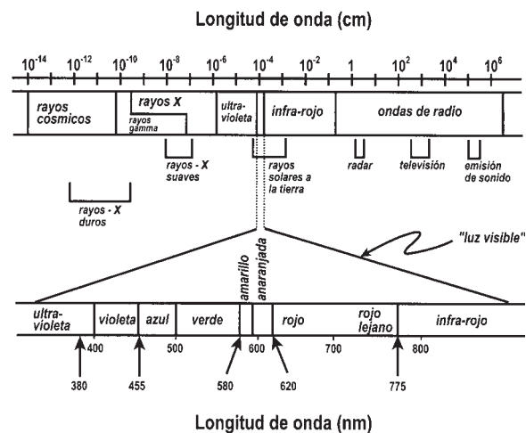
FIGURA 6.6 El espectro electromagnético. El panel superior identifica todas las posibles longitudes de onda que penetran en la estratósfera. El panel inferior muestra en detalle los componentes de la luz visible que son importantes para los procesos fisiológicos de las plantas y los organismos.
