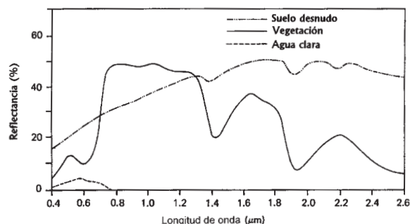
FIGURA 24.2 Patrones generalizados de respuesta espectral al suelo desnudo, la vegetación y el agua clara. (Modificado de Lillesand & Kiefer 1994.)
