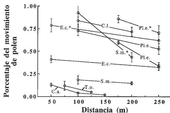
FIGURA 13.1 Desplazamiento de polen en diferentes poblaciones de árboles neotropicales de bosques continuos, en función de la distancia entre individuos receptores e individuos donantes de polen. Se presentan estimados genéticamente determinados para siete especies: Calophyllum longifolium (C.l.), Cordia alliodora (C.a.), Enterolobium cyclocarpum (E.c.), Pithecellobium elegans (Pi.e.), Platypodium elegans (Pl.e.), Spondias mombin (S.m.) y Turpinia occidentalis (T.o.; ver citas en el texto). Los estimados de flujo de genes polínicos que aparecen con un asterisco (*) son estimados de aleatorización realizados con el procedimiento Monte Carlo. Los demás estimados representan tasas de desplazamiento “evidente” de polen. Las barras representan el error estándar.
