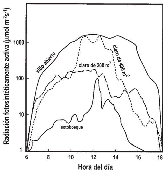
FIGURA 6.4 Patrón diario de radiación fotosintéticamente activa en la Estación Biológica La Selva, en Costa Rica, durante un día soleado en un sitio abierto, en un claro de 400 m 2 , en un claro de 200 m 2 y en un sitio en el sotobosque. Modificado de Chazdon y Fetcher (1984).
