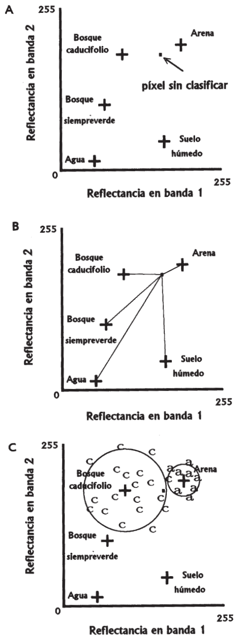
FIGURA 24.7 Ejemplo del uso del clasificador de mínima distancia a las medias. A ilustra la posición de las medias de cada clase espectral en dos bandas de una escena y la posición de un píxel cuya pertenencia se desconoce. B señala que el píxel desconocido se asignaría a la clase “arena”, por ser esta la clase cuya media le queda más cercana. Sin embargo, al observar en C las posiciones de los píxeles contenidos en los campos de entrenamiento de las clases “arena” (a) y “bosque caducifolio” (c) se ve que es más apropiado asignar el píxel desconocido a la clase “bosque caducifolio”, por estar localizado dentro del círculo que define una desviación estándar de esa nube de píxeles.
