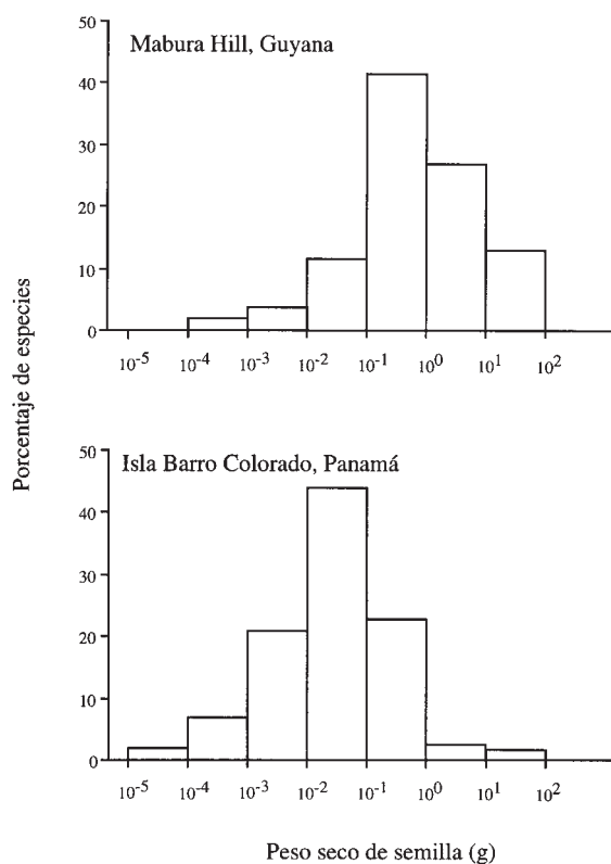
FIGURA 15.1 Variación en el tamaño de las semillas en dos bosques neotropicales, Mabura Hill en Guyana (Hammond & Brown 1995) y la Isla de Barro Colorado, en Panamá (Foster 1982). Como consecuencia de su tamaño, en Guyana la mayoría de las especies, sobre todo de árboles, es dispersada por mamíferos (Hammond et al. 1996), en cambio, en la Isla de Barro Colorado esa proporción es mucho menor (Hammond & Brown 1995).
