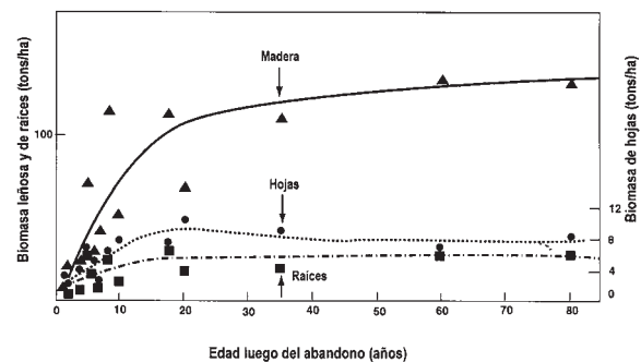
FIGURA 23.6 Biomasa de hojas, raíces y tejido leñoso (ramas, troncos), expresada en toneladas por hectárea y en función del tiempo de abandono del sitio, en diferentes localidades del trópico húmedo. Modificado de Brown y Lugo (1990a).
