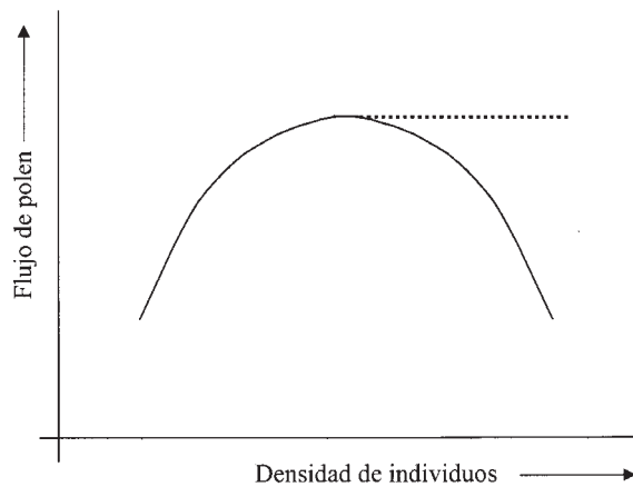
FIGURA 20.3 Flujo de polen, expresado en términos de la distancia entre la planta donante y la planta receptora, y generado por un polinizador generalista (línea continua) o por uno especialista (línea punteada) en función de la densidad de individuos en flor.
