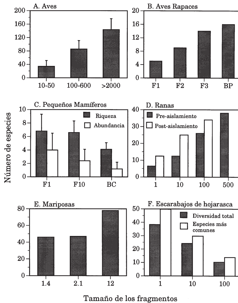
FIGURA 22.3 Relación entre el área del fragmento y el número de especies en varios grupos taxonómicos. A. Número de especies de aves ( \pm desviación estándar) en bosques nublados de los Andes de Colombia, como función del tamaño de los fragmentos (en ha) (modificado de Kattan & Alvarez-López 1996). B. Número de aves rapaces de bosque de la Guayana Francesa como función del grado de fragmentación del paisaje; F1, paisaje fragmentado con cobertura de bosque <33 %; F2, paisaje con cobertura de bosque 33-66 %; F3, paisaje con cobertura de bosque >66 %; BP, bosque primario (modificado de Jullien & Thiollay 1996). C. Riqueza, en número de especies por hectárea y abundancia, en número de capturas por hectárea, de pequeños mamíferos terrestres de la Amazonia central, para fragmentos de 1 ha (F1), 10 ha (F10) y bosque continuo (BC) (modificado de Malcolm 1997). D. Número de especies de ranas de la Amazonia central en parches de bosque de 1, 10, 100 y 500 ha antes y después del aislamiento (modificado de Tocher et al. 1997). E. Número de especies de mariposas en fragmentos de bosque urbanos (área en ha) en el sureste de Brasil (modificado de Rodrigues et al. 1993); a pesar del pequeño tamaño, estos fragmentos tienen una alta diversidad de especies. F. Pérdida de escarabajos de la hojarasca (expresado como porcentaje de especies desaparecidas) como función del área del fragmento (en ha), en bosques de la Amazonia central (modificado de Didham et al. 1998).
