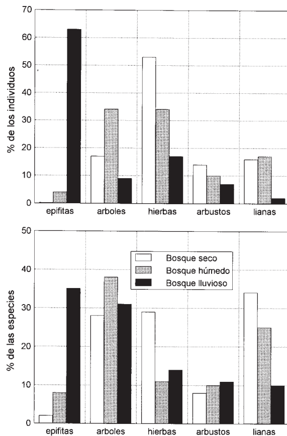
FIGURA 12.1 Importancia relativa de varias formas de crecimiento en tres bosques ecuatorianos –bosque seco (Capera), bosque húmedo (Jauneche) y bosque lluvioso (Río Palenque)– ubicados a lo largo de un gradiente de precipitación. El cuadro superior muestra el porcentaje de individuos y el inferior, el porcentaje de especies de cada forma de crecimiento (modificado de Gentry & Dodson 1987a).
