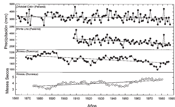
FIGURA 7.5 En los paneles superiores, precipitación anual en las estaciones meteorológicas de “Cristóbal Colón” y “Monte Lirio” en la costa Caribe e interior del istmo de Panamá, respectivamente. Las regresiones son estadísticamente significativas tanto para Colón ( P < 0.05 ) como para Monte Lirio ( P < 0.001 ). Solo para las precipitaciones en Monte Lirio ( P < 0.001 ) la línea tiene una pendiente significativamente distinta de cero (Cristóbal Colón: P = 0.36 ). Datos tomados de Windsor (1990). En los dos paneles inferiores, precipitación anual y número de meses secos ( < 100 mm) en la estación de Roseau, Dominica (1865-1989). Las regresiones son estadísticamente significativas tanto para la precipitación anual ( P < 0.001 ) como para los meses secos ( P < 0.001 ). Tanto para las precipitaciones como para los meses secos, las líneas tienen una pendiente significativamente distinta de cero ( P < 0.001 ). Modificado a partir de Walsh (1996).
