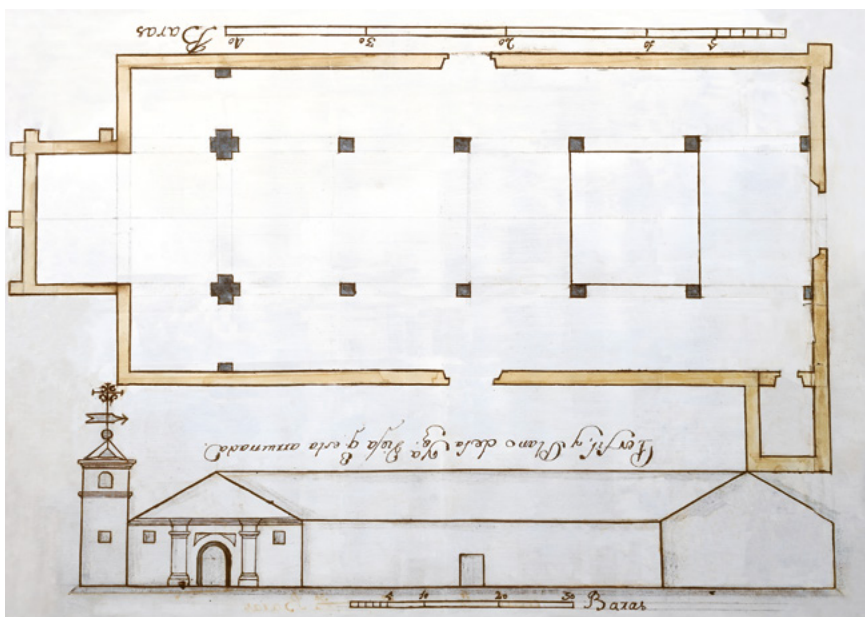
Planta, alzado y sección transversal de la antigua catedral de Santa Marta (1767). Archivo General de Indias, MP-PANAMA, 175.
