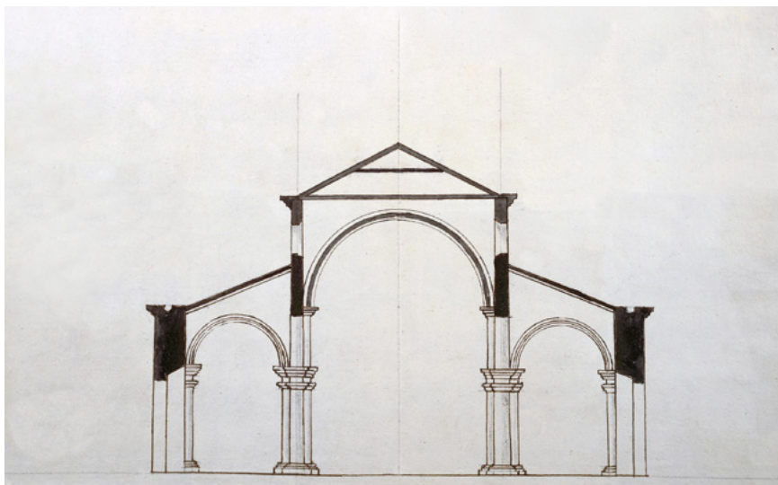
Planta, alzado y sección transversal de la antigua catedral de Santa Marta (1767). Archivo General de Indias, MP-PANAMA, 175.
