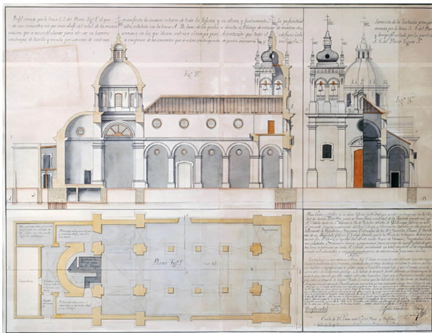
Plano, vistas y perfiles de la Iglesia Catedral de Santa Marta (1767). Archivo General de Indias, MP-PANAMA, 176.
