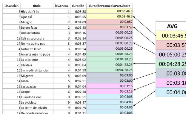
Figura 6.9. Ejemplo de agrupamiento de filas con utilizando cláusula GROUP BY
