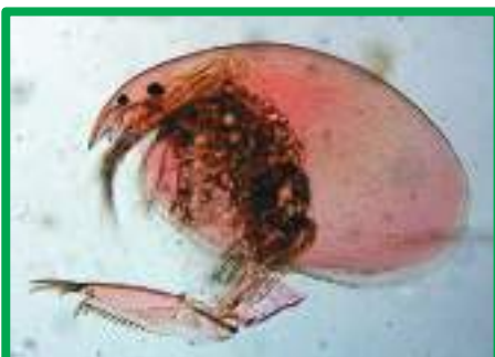
Oxyurella longicaudis
