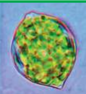
Lepocinclis fusiformis
