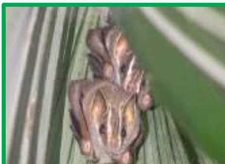
Uroderma bilobatum
